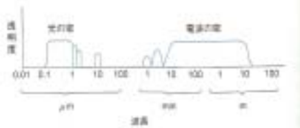
●図 5.2 電波の波、光の波
